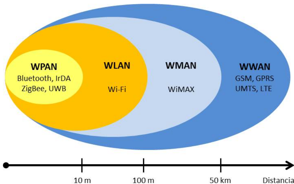
Fig. 1.1 Clasificación de las redes inalámbricas
