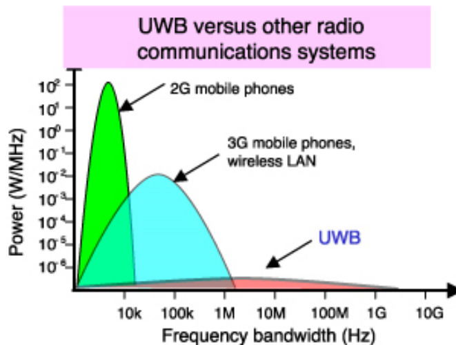
Figure 1.5 Utilización del ancho de banda frecuencial y consumo de energía por la tecnología UWB.
