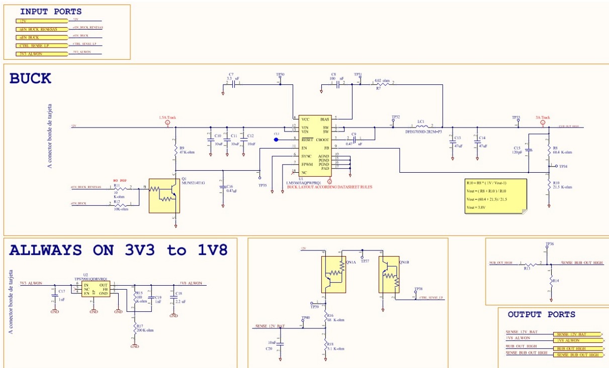
Fig. 4. Esquemático de PCB.
